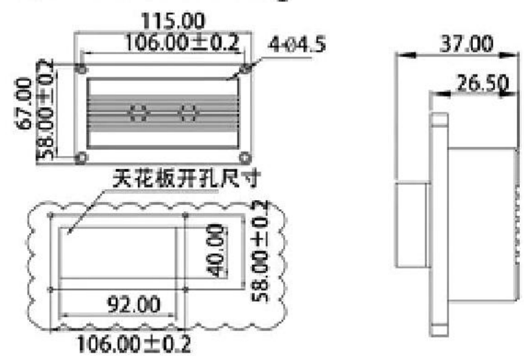
【室内麦克风 HLD-MIC600】重量：0.4kg
