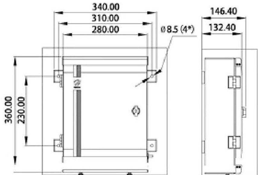
【串行数据采集单元 HLD-DAU600】重量：8.0kg
