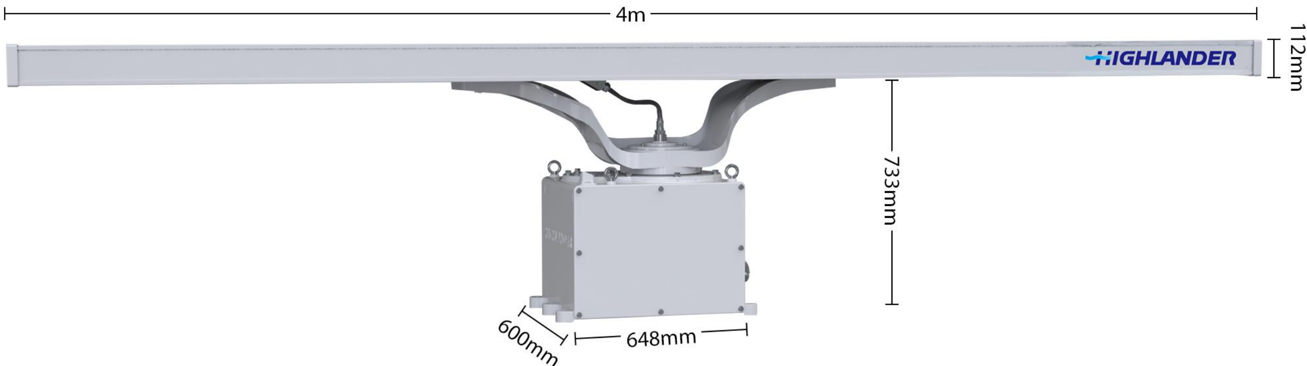
【HLD-AT112+TU225 S-band radar】 186kg
